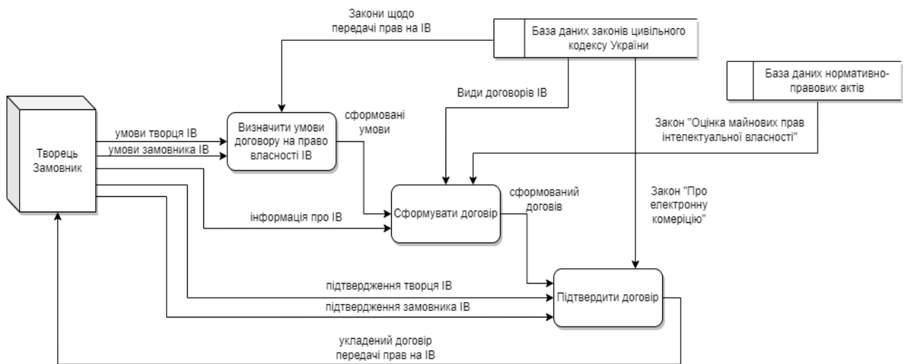
Рис. 1. Діаграма потоків даних щодо формування договору купівлі-продажу об'єктів права інтелектуальної власності та передачі прав власності на продукт з урахуванням зовнішніх чинників впливу
